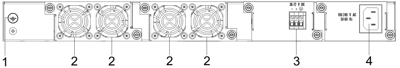
Рисунок 21 – Задняя панель MES5312, MES5324A, MES5332A
