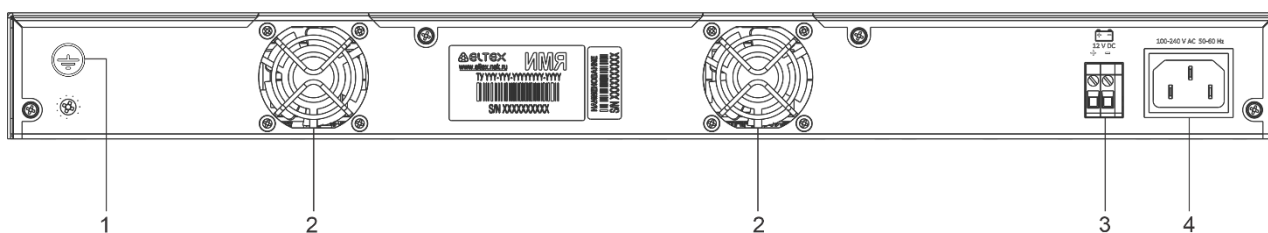
Рисунок 17 – Задняя панель MES2300B-48
