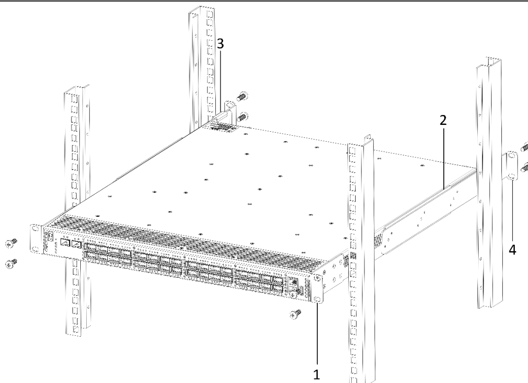
Рисунок 52 – Установка устройства MES5500-32 в стойку
