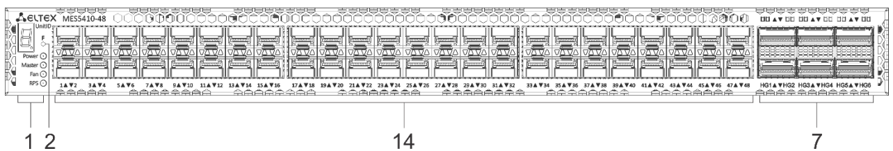
Рисунок 13 – Передняя панель MES5410-48
