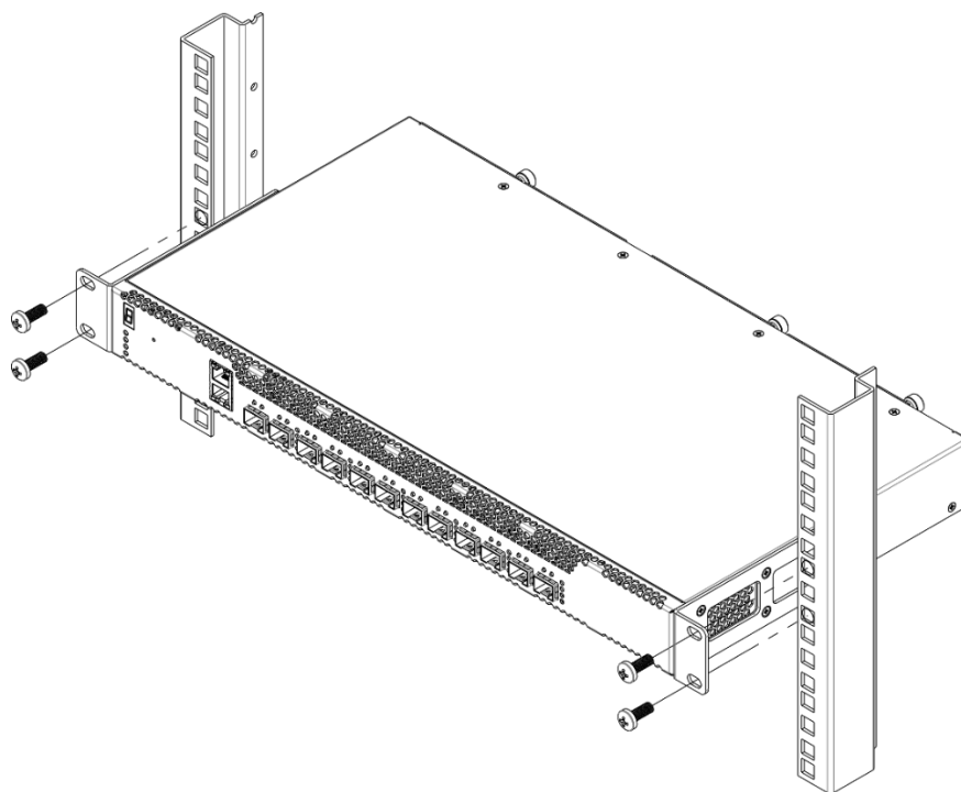
Рисунок 51 – Установка устройства в стойку
