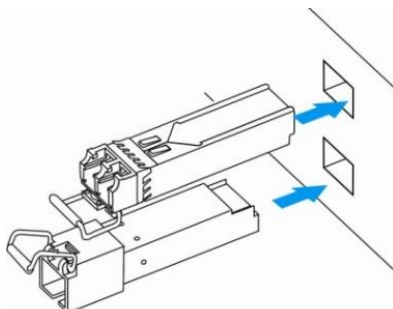
Рисунок 55 – Установка SFP-трансиверов
