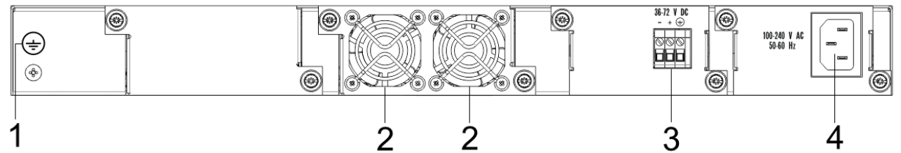
Рисунок 22 – Задняя панель MES5316A
