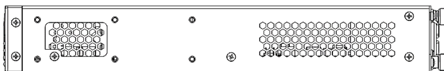
Рисунок 35 – Правая боковая панель MES5316A, MES5324A, MES5332A
