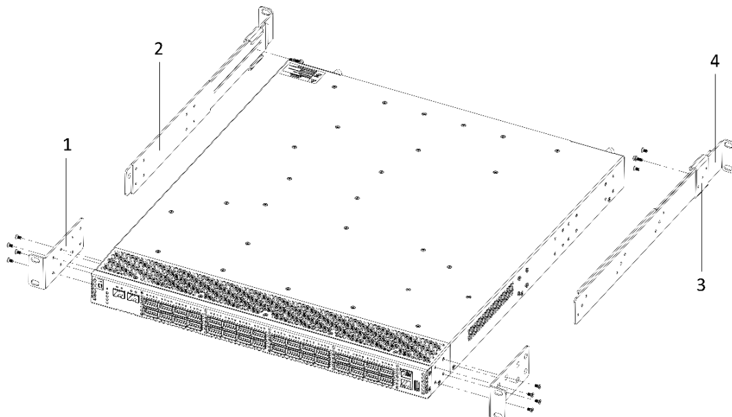
Рисунок 50 – Вариант крепления кронштейнов для MES5410-48, MES5500-32
