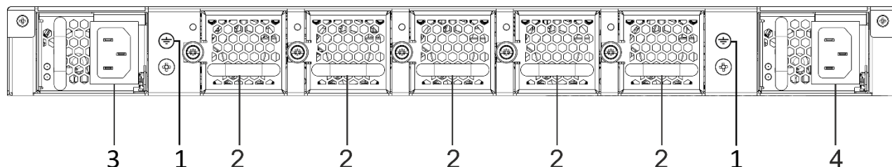
Рисунок 26 – Задняя панель MES5500-32
