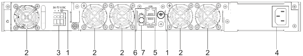
Рисунок 24 – Задняя панель MES5400-48
