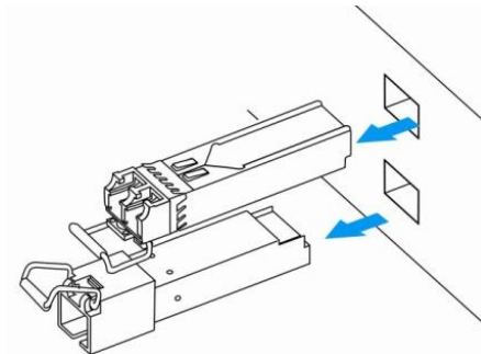
Рисунок 58 – Извлечение SFP-трансиверов
