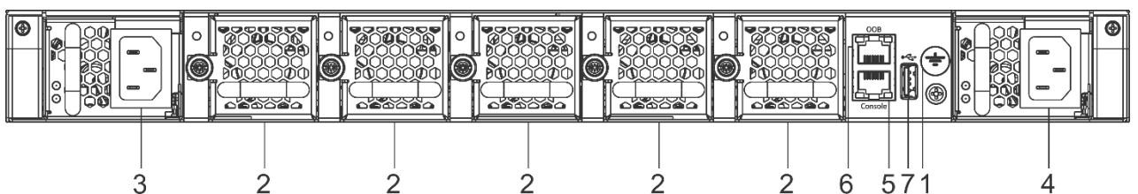
Рисунок 25 – Задняя панель MES5410-48
