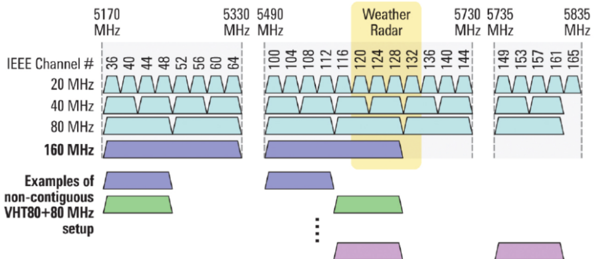
Рисунок 6 – Каналы, используемые в диапазоне 5 ГГц при ширине канала 20, 40, 80 МГц
